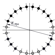
DN 700-800
