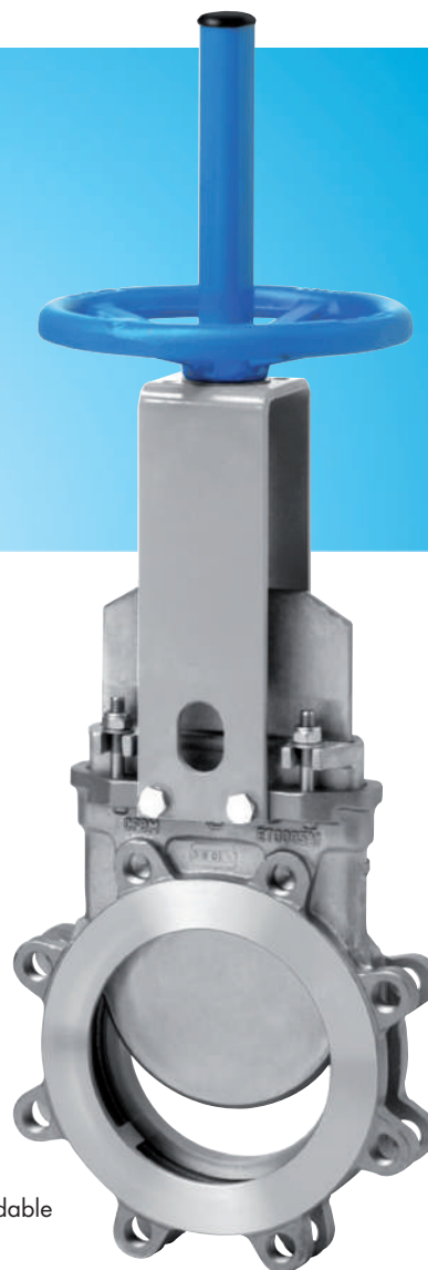
ET Unidireccional MSS SP-81 DN 50 – DN 900 acero inoxidable
