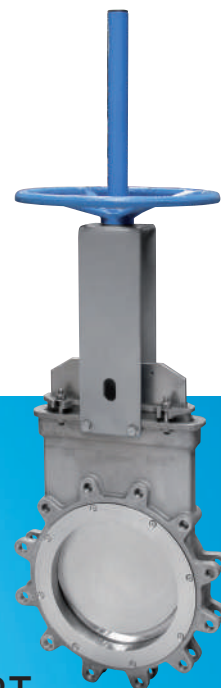
BT Bidireccional MSS SP-81 DN 50 – DN 900 acero inoxidable
